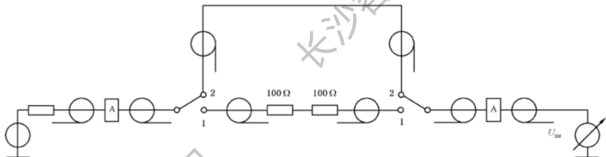
b) 验证耦合/去耦装置 Z_{0c} 的配置原理图
