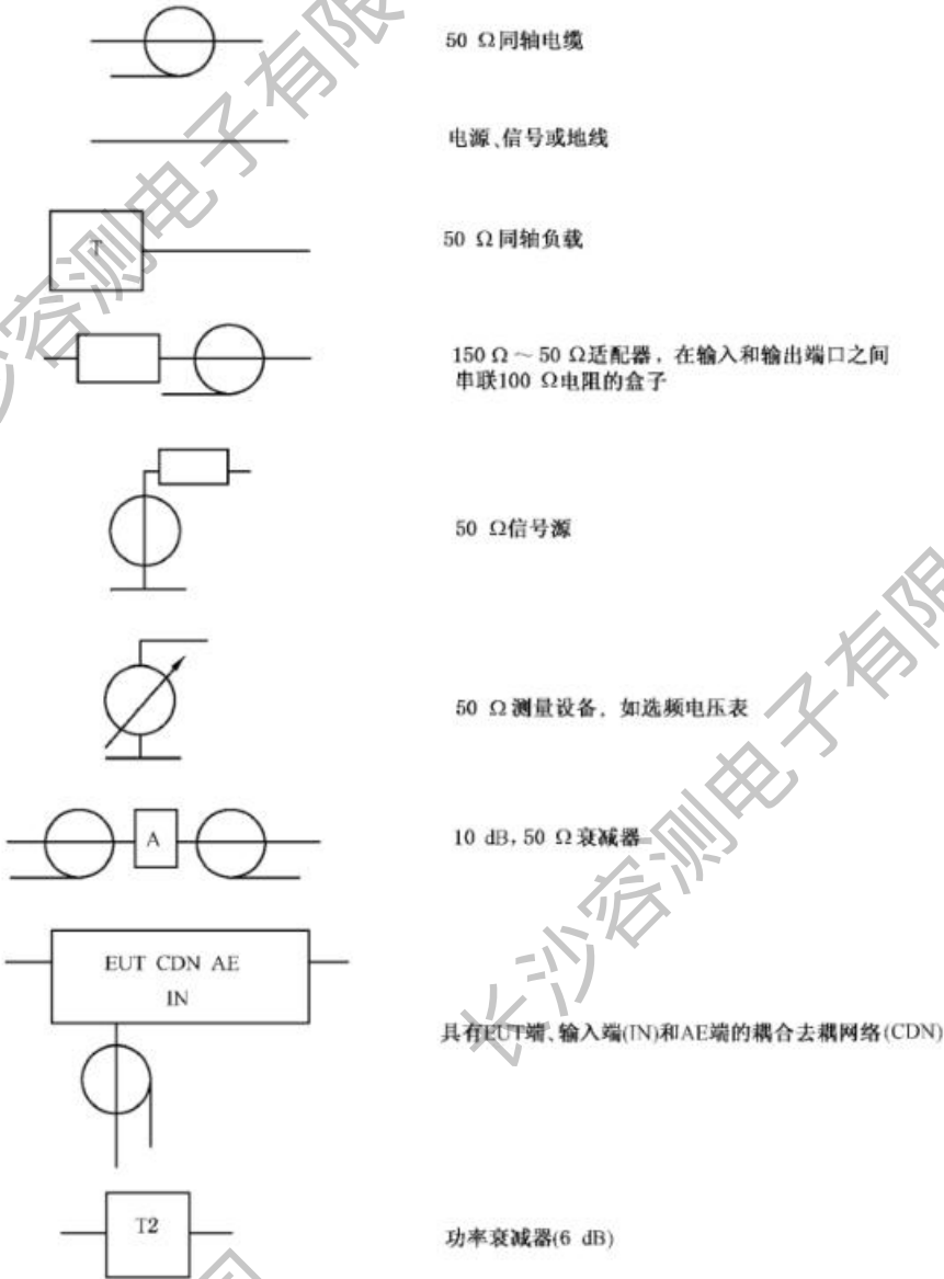
a) 用于测量配置图中的符号清单
